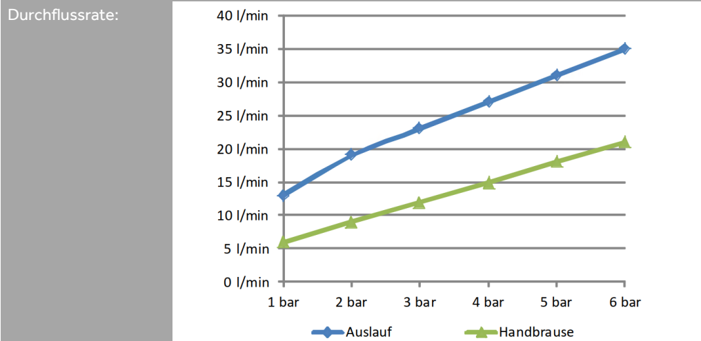
2-Stufige Eco-Kartusche mit Wassersparfunktion
